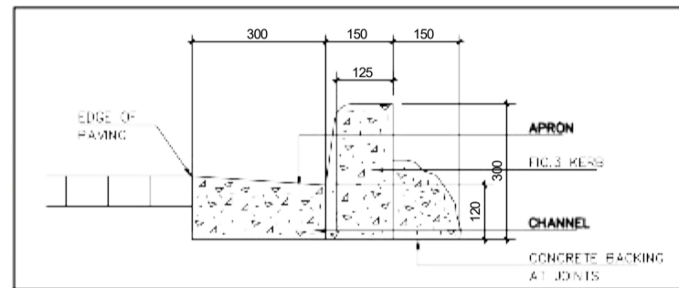
UNMOUNTABLE KERB N.T.S
