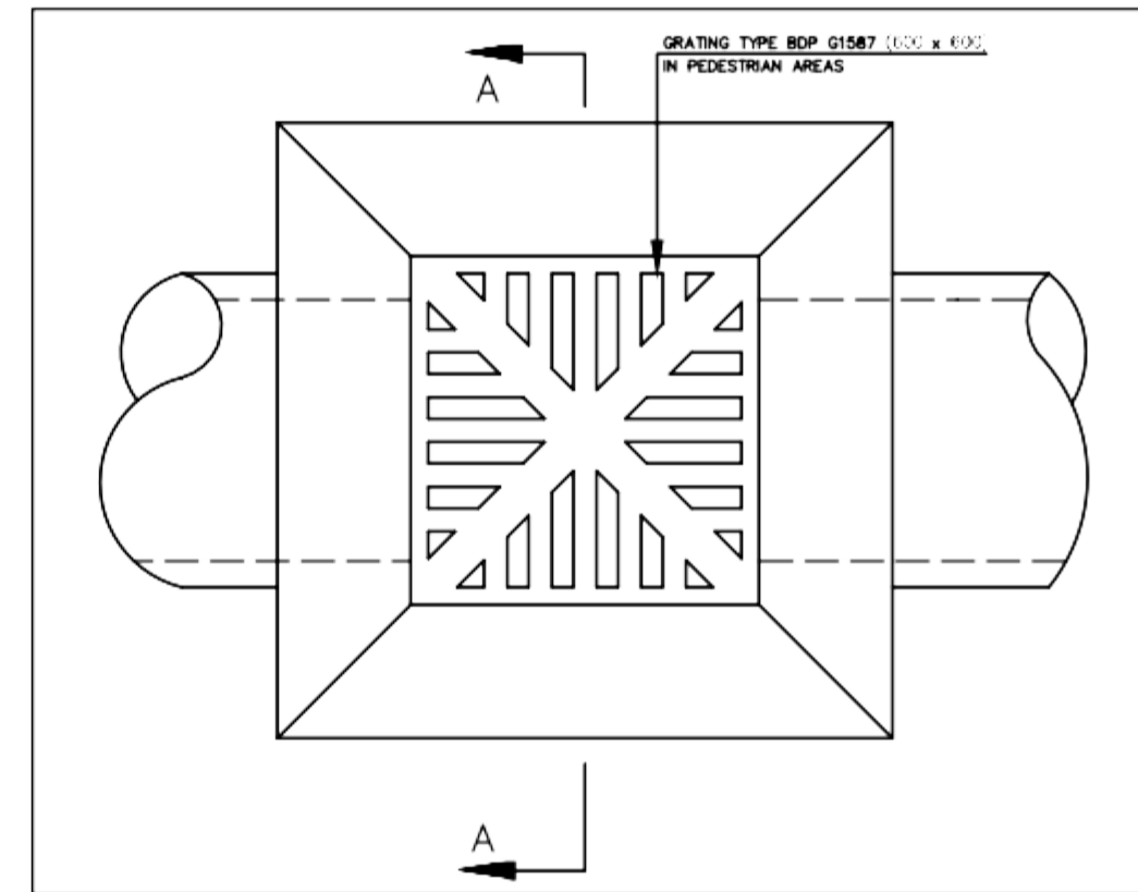
GRID INLET N.T.S
