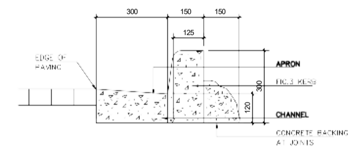
UNMOUNTABLE KERB N.T.S
