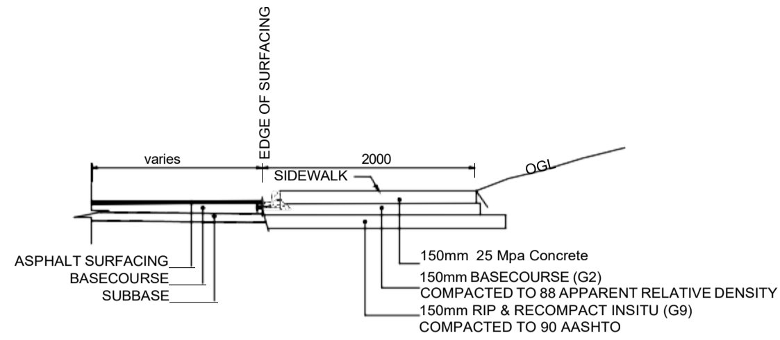
SIDEWALK CROSS SECTION N.T.S
